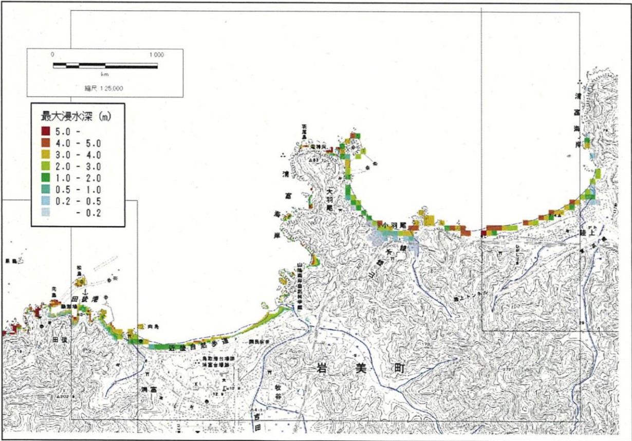
最大浸水深図（範囲 3 0）
