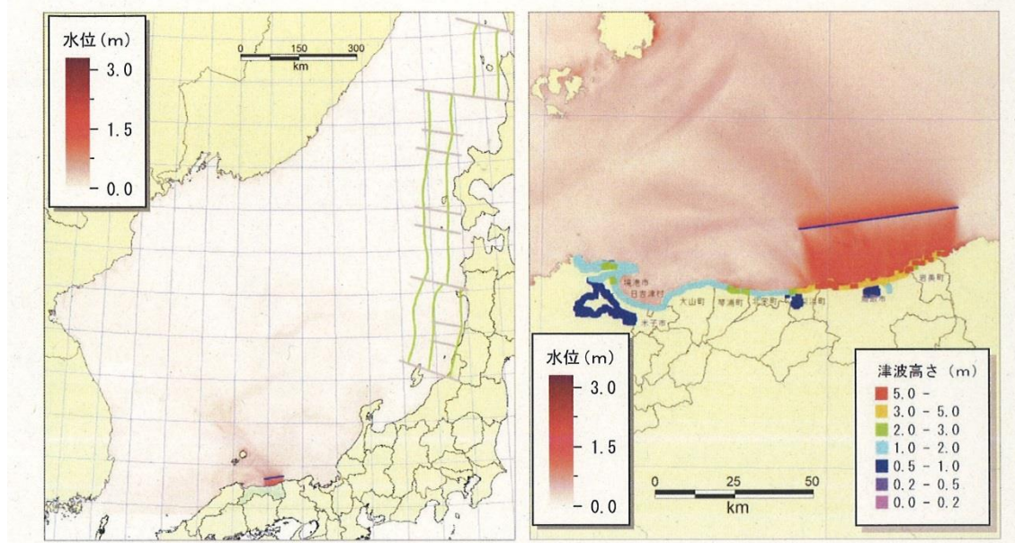
図 4.1.5 津波の計算結果（海岸の津波の高さ）【鳥取沖東部断層（北上がり）】
