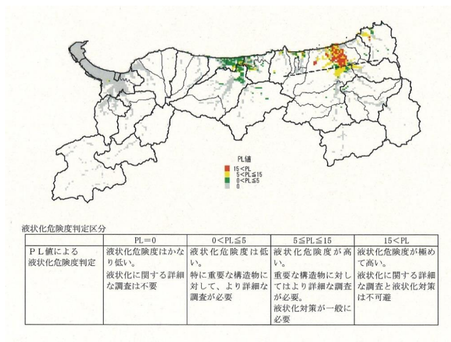
図 4.1.3 鹿野・吉岡断層による地震 液状化危険度分布
