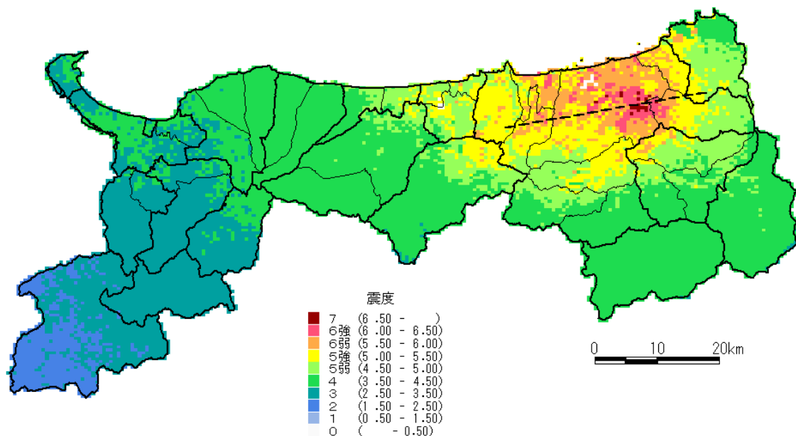
図4.1.1 鹿野・吉岡断層による地震の予測結果
