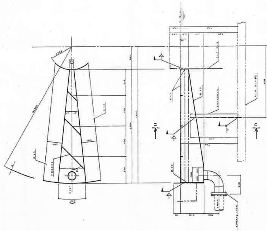
スチールボックス断面図
