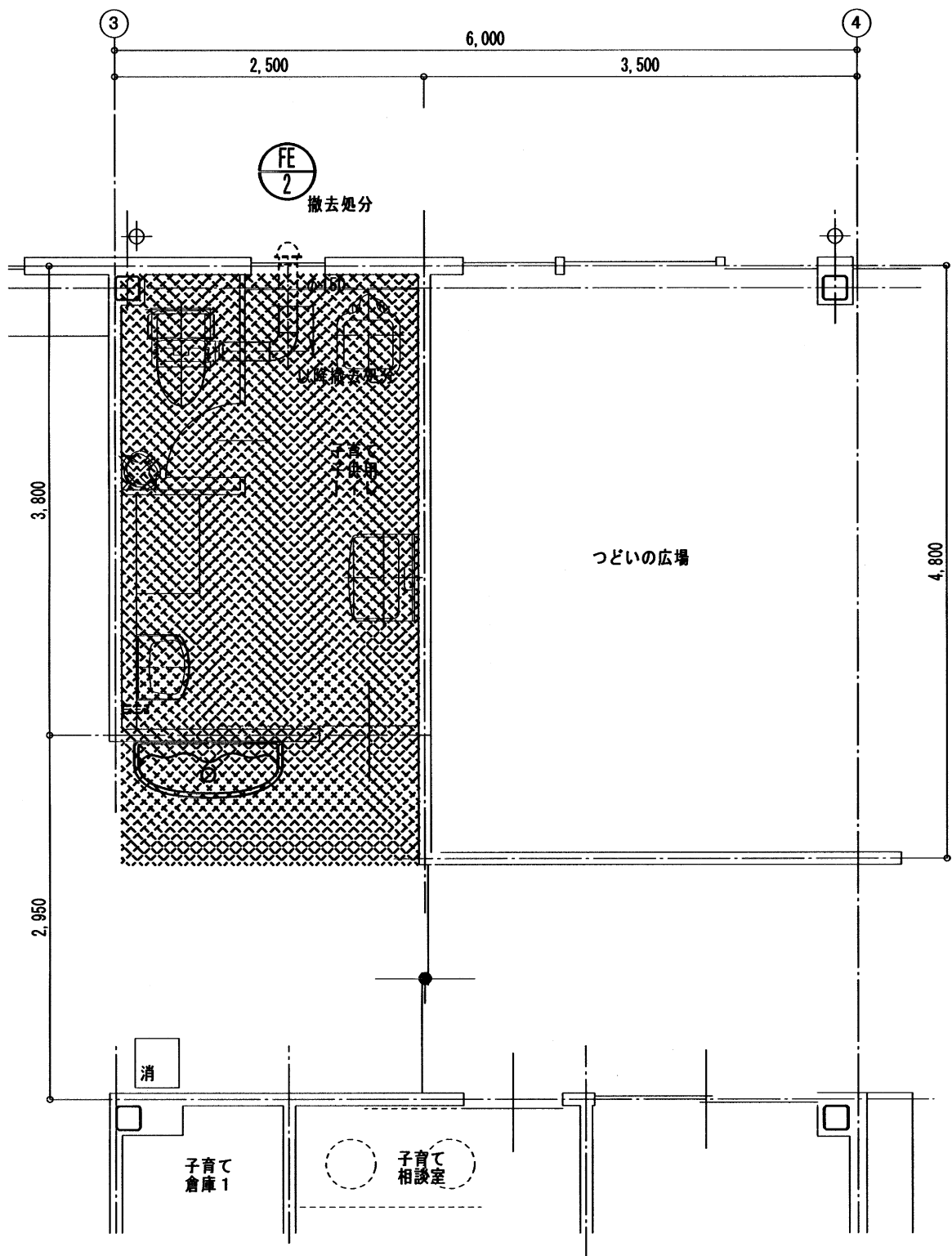
撤去参考図 S=1/50 トイレ天井解体、廃材処分は建築工事
