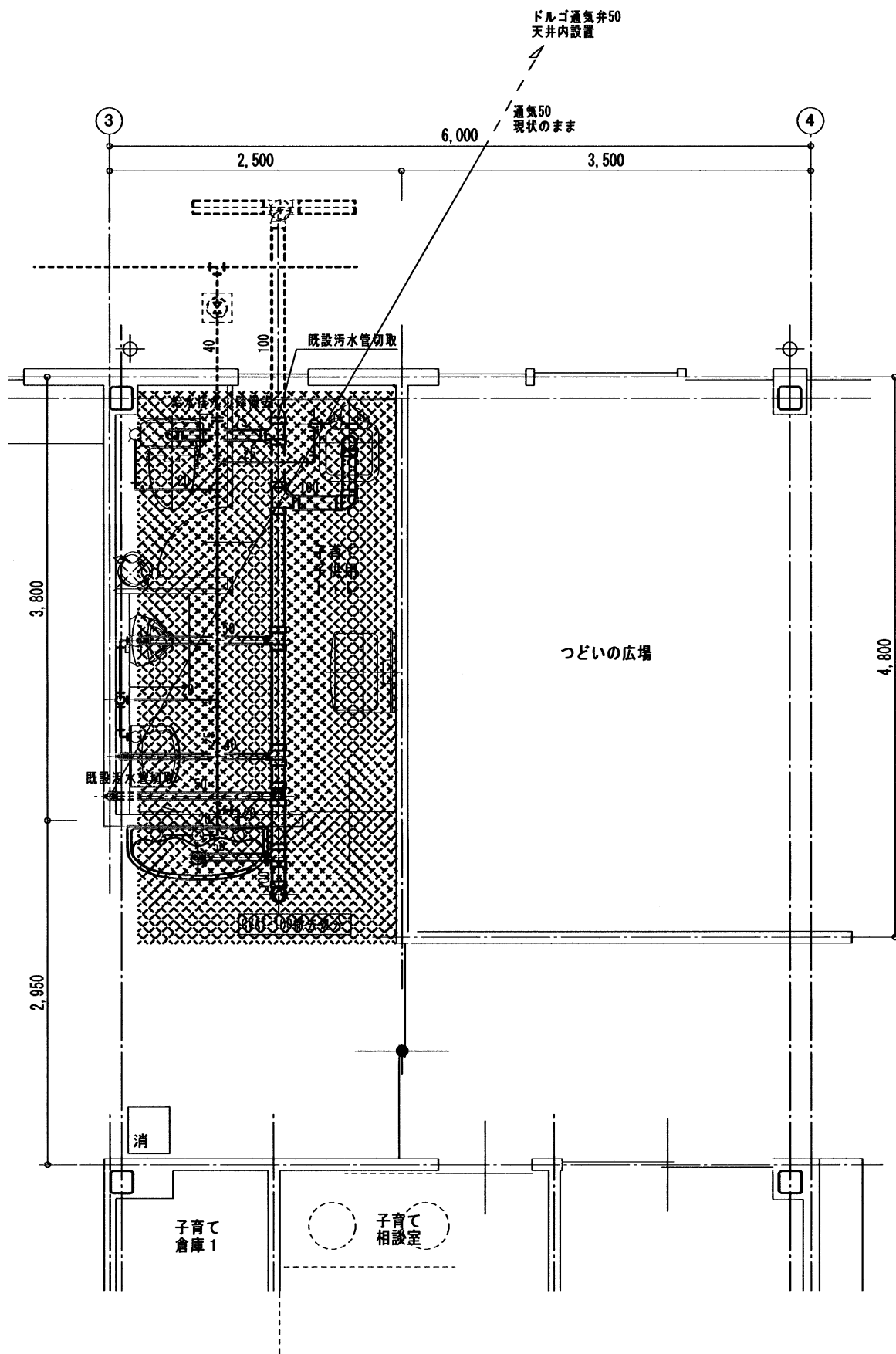
撤去参考図 S=1/50
