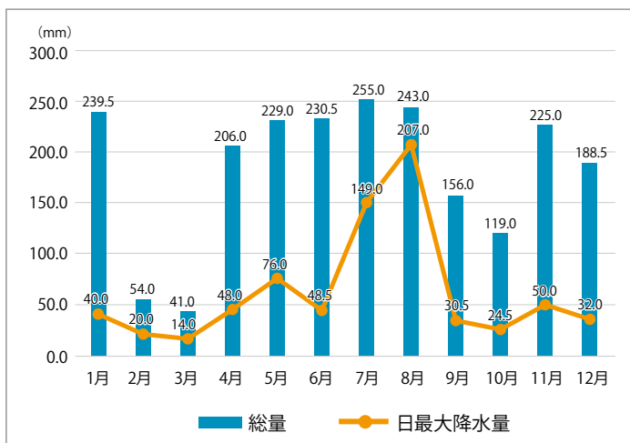
降水量
