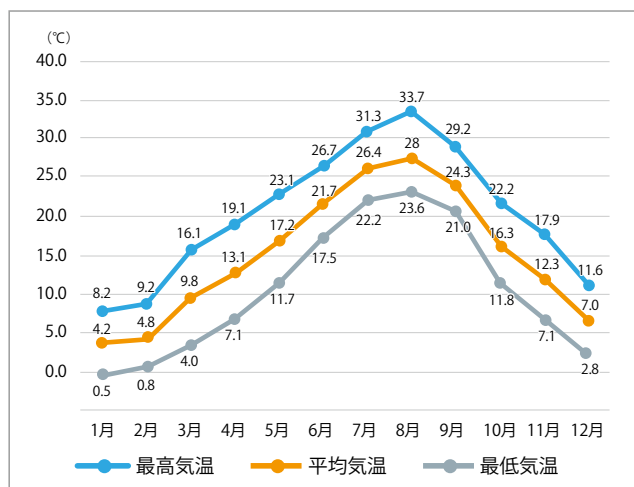
気温
