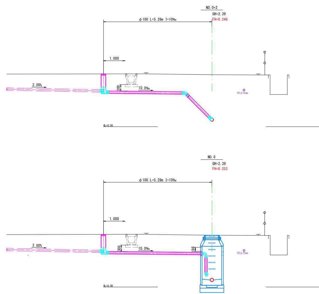
管路横断面図(ペーロケ) S=1:50
