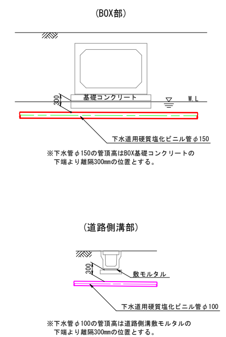
下越し拡大図 S=1:50
