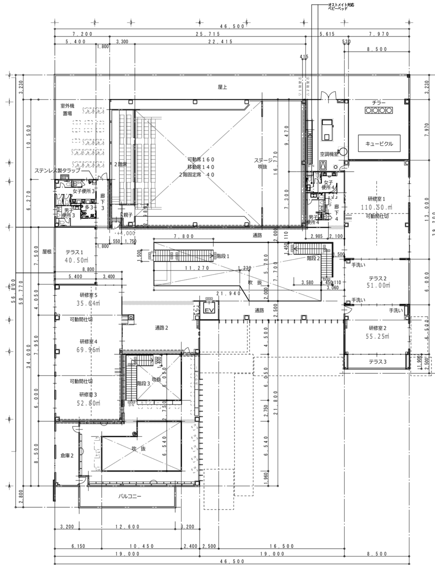
2階平面図
