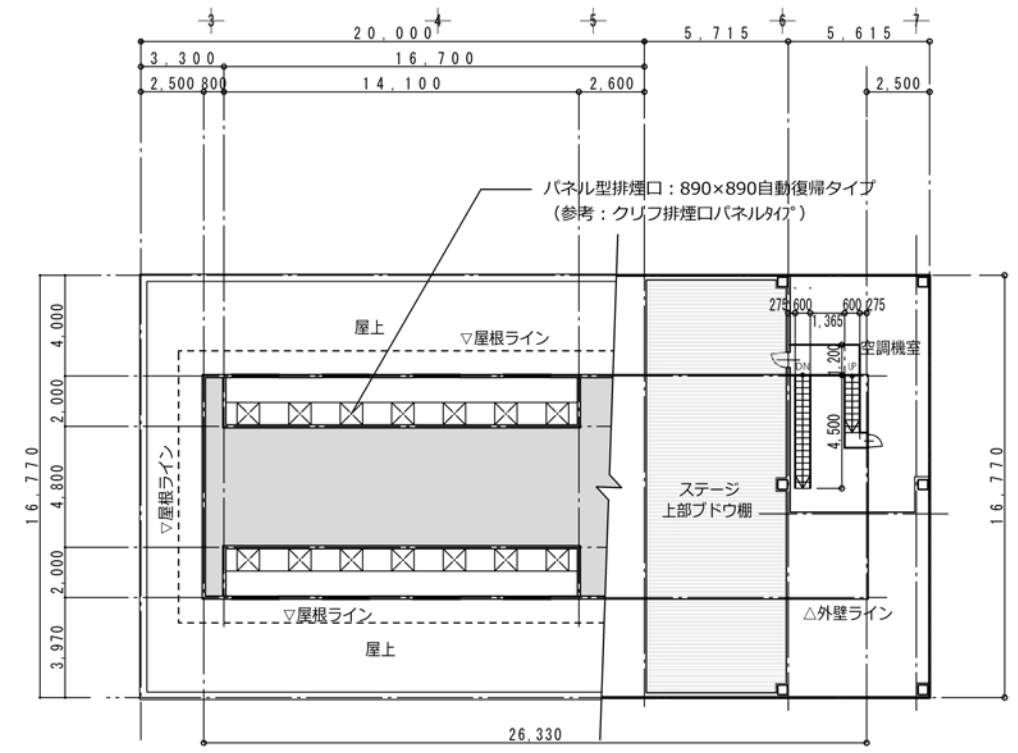
排煙口平面図
