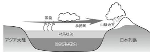
図2：山陰海岸ジオパークに雪が降るしくみ
